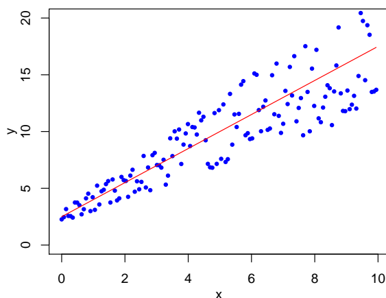
Heteroscedastic Data
